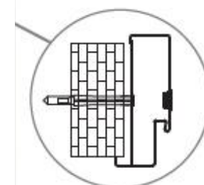
otwór montażowy kotwy w centrum profilu na pierś ościeżnicy
