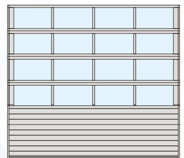
BRAMA Z PANELAMI Z SEKCJĄ ALUMINIOWĄ PRZESZKLONĄ
