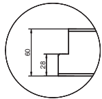
Przekrój skrzydła EI 2 60 F3, F4
