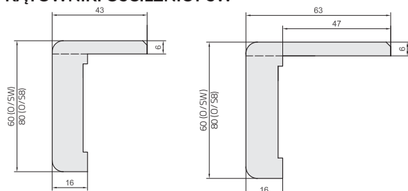
Element narożny ościeżnicy SW kątownik standard
