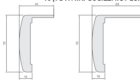
Element narożny ościeżnicy LUX kątownik standard
