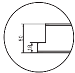
Przekrój skrzydła EI 2 30 F1, F2
