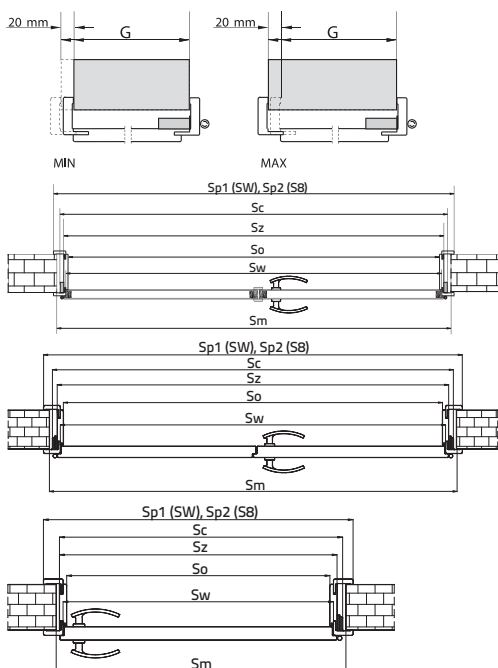
WYMIARY OŚCIEŻNIC REGULOWANYCH SW/S8 DO DRZWI DWUSKRZYDŁOWYCH W TECHNOLOGII STANDARD, SOFT ORAZ TECHNOLOGII RAMA SOFT WYMIARY STANDARDOWE
