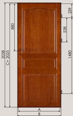
Wymiary skrzydeł przylgowych
